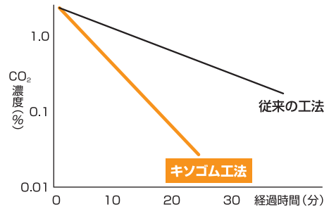
■床下換気測定試験 (JIS A 1406)
