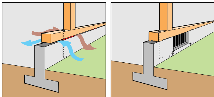
■キソゴム工法
